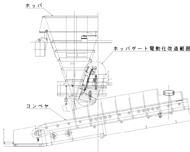
ホッパゲート電動化計画図 参考図
