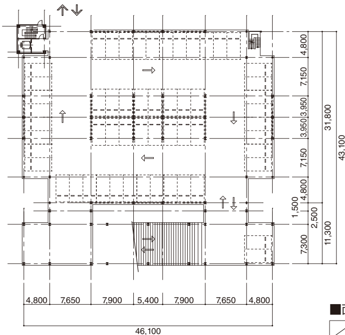
■1階平面図
