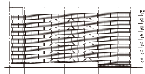
■立面図
